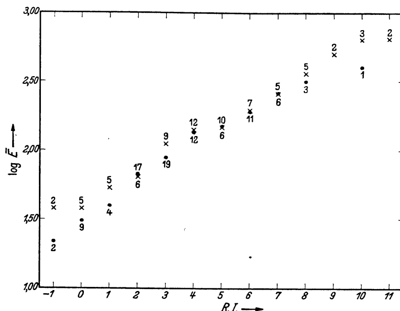
Abb. 4. Zusammenhang zwischen Rowland-Intensität und Äquivalentbreiten für Photosphärenlinien (•) und Fleckenlinien (×).
