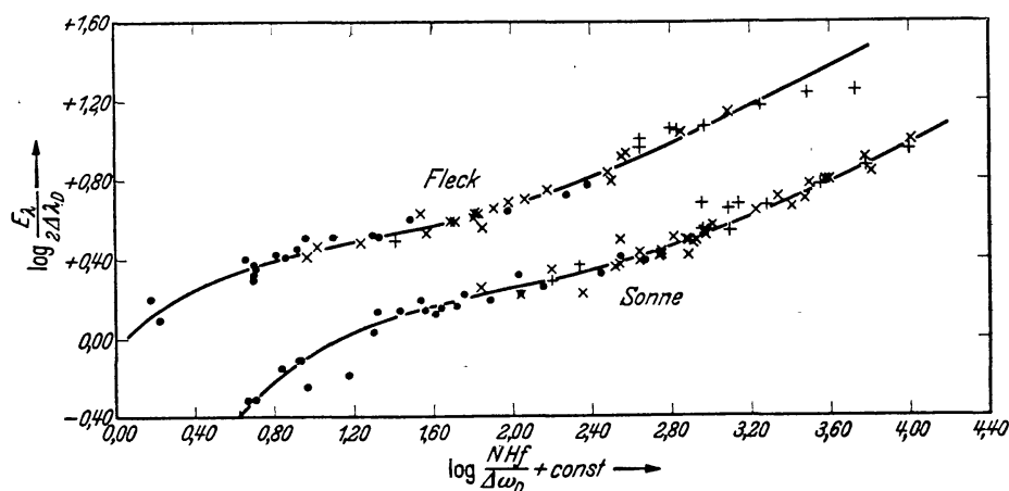
Abb. 10. WK für Fleck und Photosphäre.
