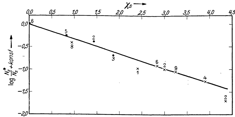
Abb. 11. \log N_s^*/N_s als Funktion des Anregungspotentials \chi_s . • Ti-Linien, \times Fe-Linien.
