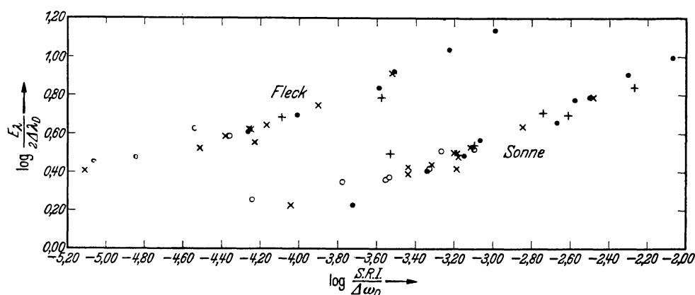
Abb. 7. Aus Fe-Linien gewonnene WK für Photosphäre und Fleck.
