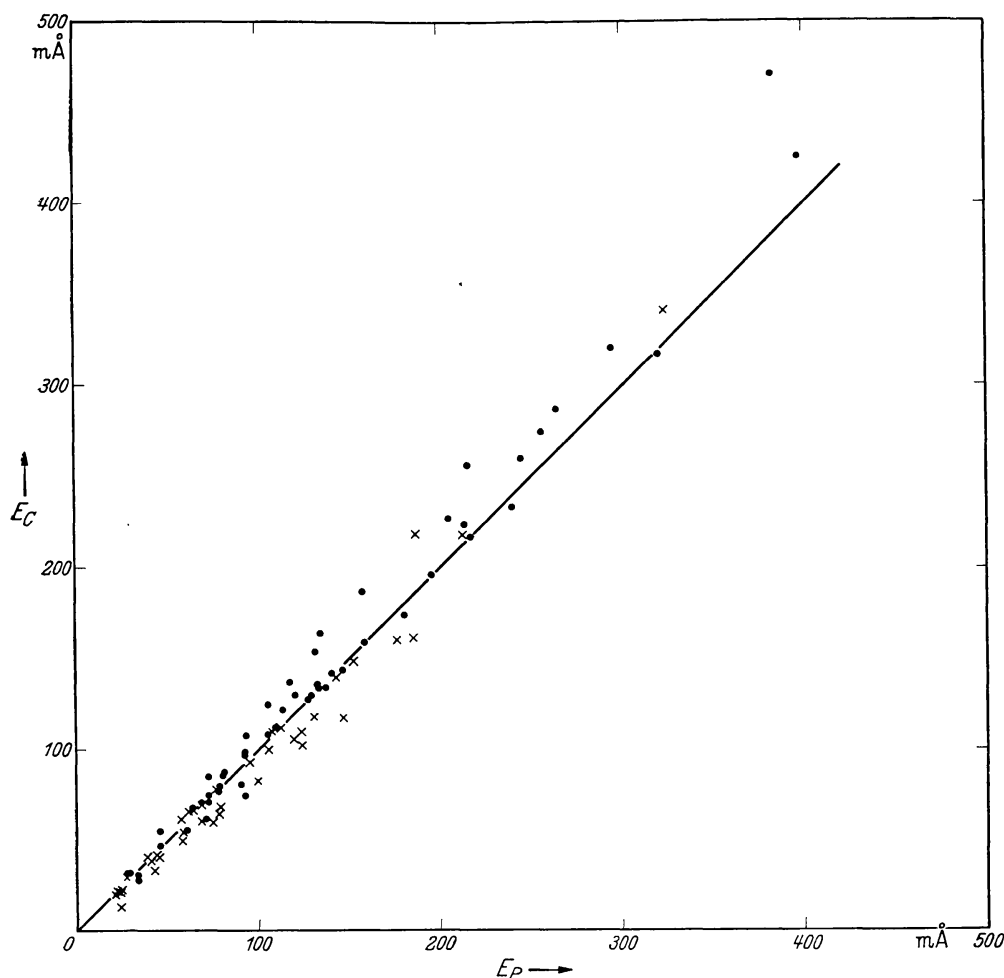
Abb. 3. Zusammenhang zwischen den in Potsdam ( E_P ) und Canberra ( E_C ) gemessenen Äquivalentbreiten von Fraunhofer-Linien. Die Werte von E_C sind teils aus Linienkonturen (•) und teils aus Restintensitäten (×) gewonnen worden.
