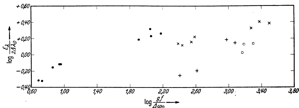
Abb. 5. Relative Verschiebungen einzelner Ti-Multipletts im WK-Diagramm.
