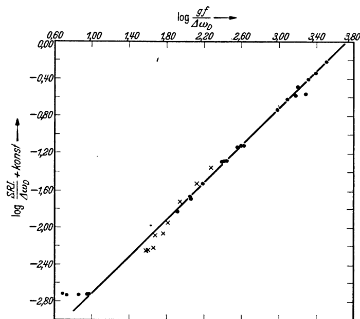
Abb. 8. Zusammenhang zwischen Summenregelintensitäten und gf -Werten für Ti-Multipletts (●) und ein Fe-Multiplett (×).
