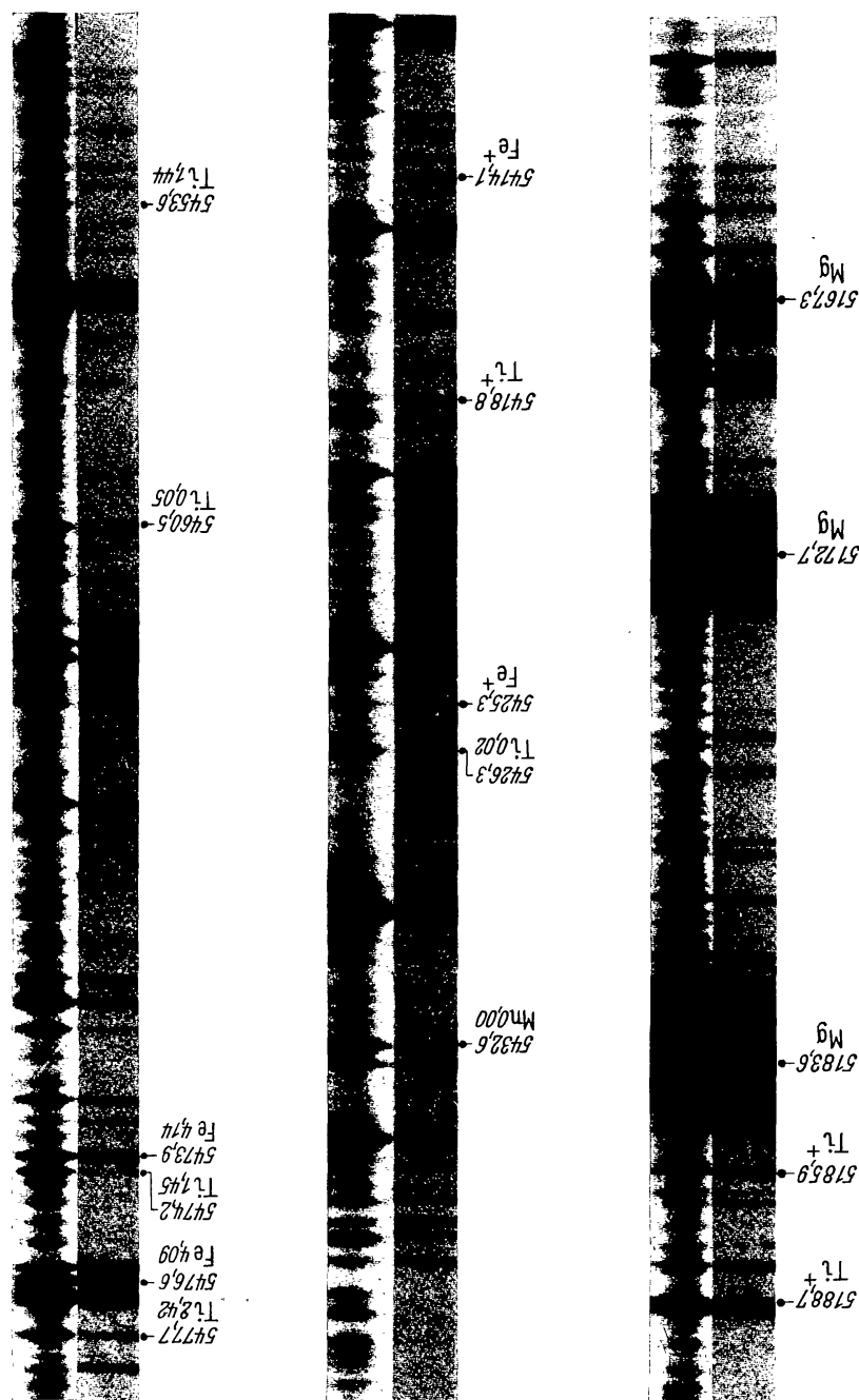
Abb. 12. Ausschnitte von Flecken- und Photosphärenspektren.
