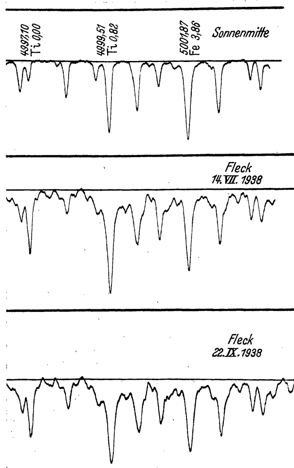
Abb. 2. Registrierkurven eines Photosphärenspektrums und zweier Fleckenspektren. Die kräftigen horizontalen Graden stellen die jeweiligen Nullmarken (vollkommene Dunkelheit) der Registrierkurven dar. Für drei Linien sind die Wellenlängen, Elementsymbole und Anregungspotentiale in Volt angegeben.
