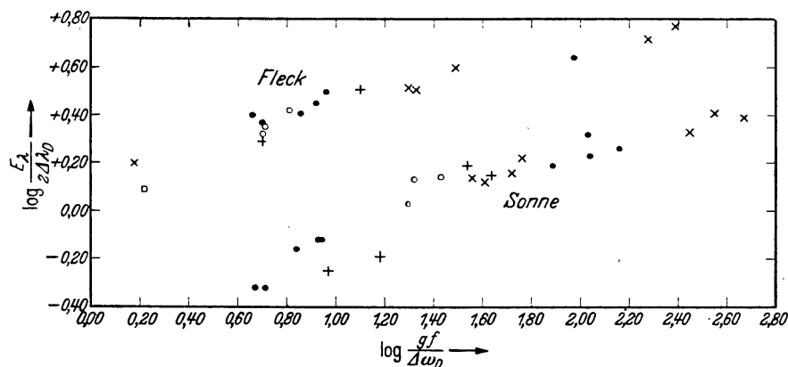
Abb. 6. Aus Ti-Linien gewonnene WK für Photosphäre und Fleck.
