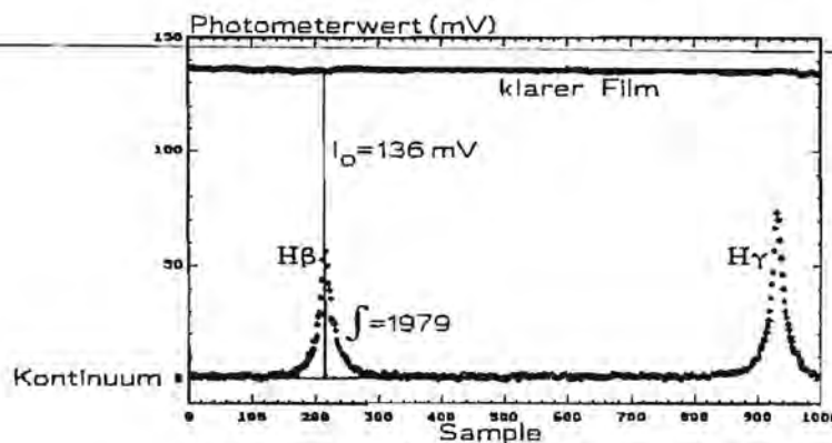
Abb.3 Fotografisches Spektrum \alpha Lyr Dispersion im Scan = 1,36 Sample/ \text{\AA}
